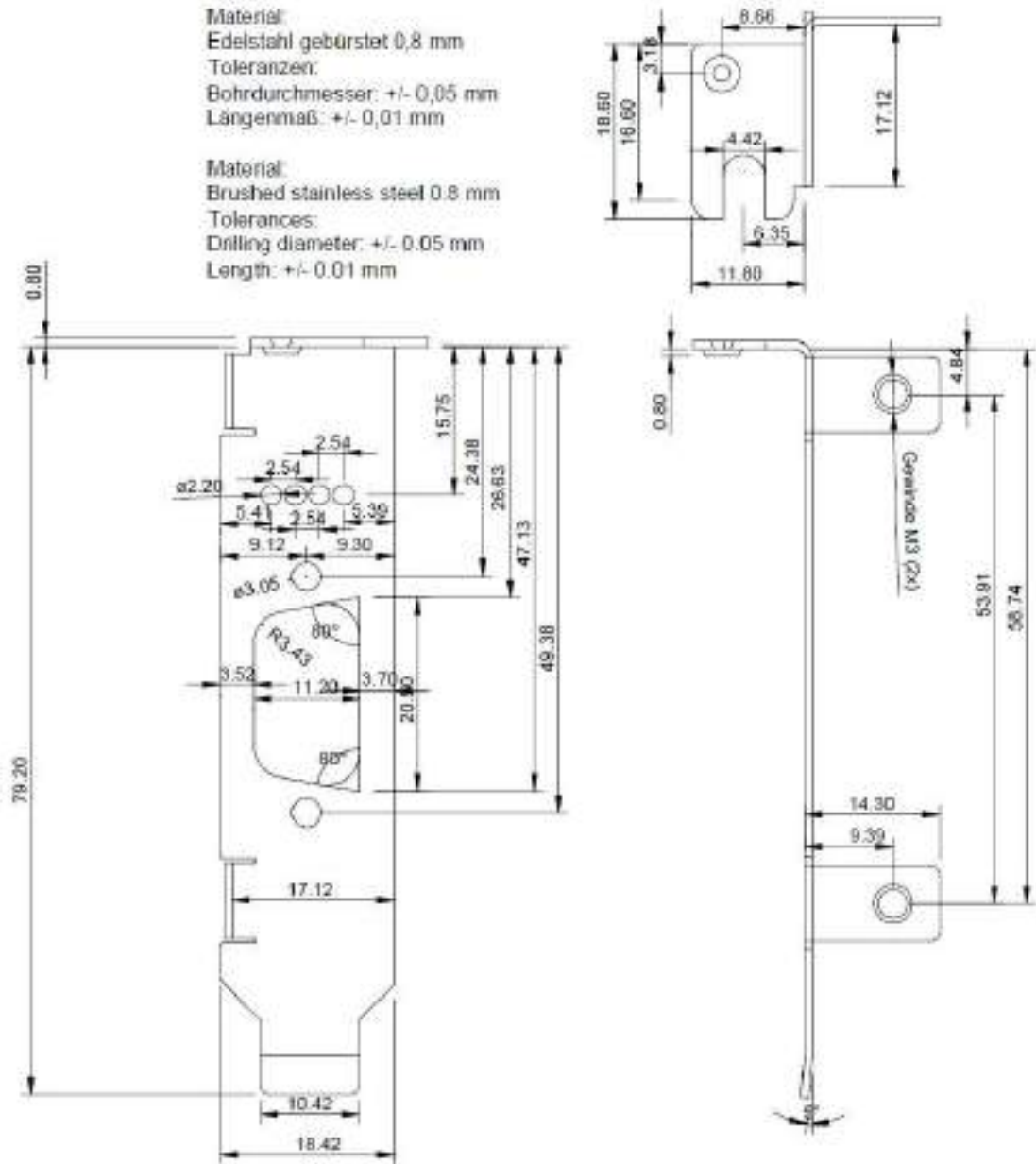
Figure 105: Blende für CIFX 70E-DP, CIFX 70E-DPMR
